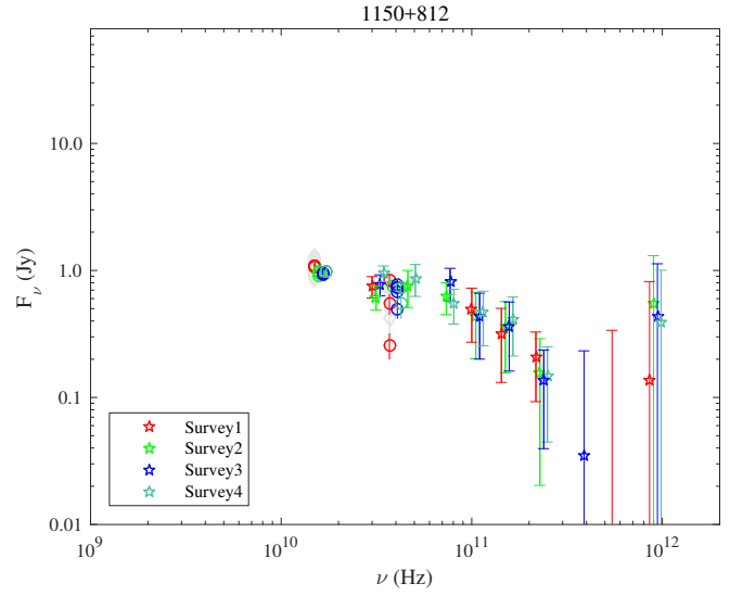
Fig. A.52. 1150+812.
