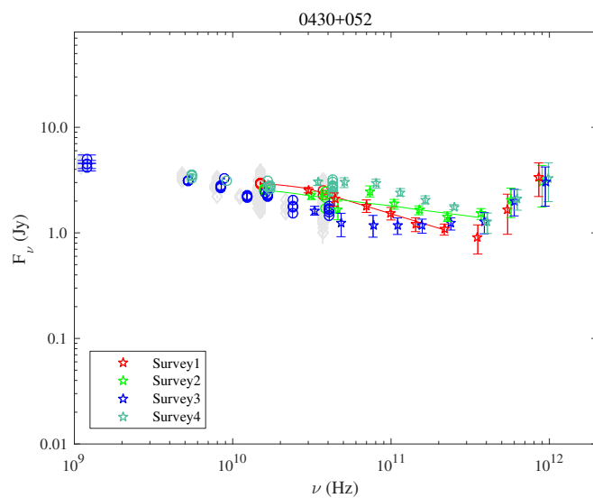
Fig. A.22. 0430+052.
