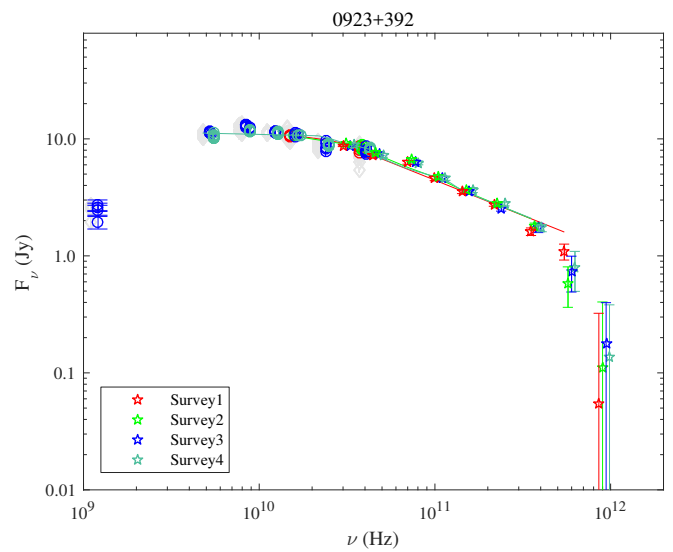
Fig. A.44. 0923+392.
