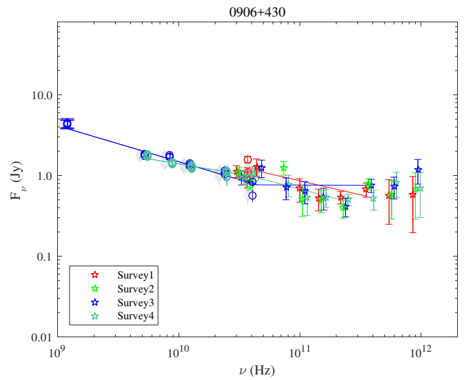
Fig. A.42. 0906+430.
