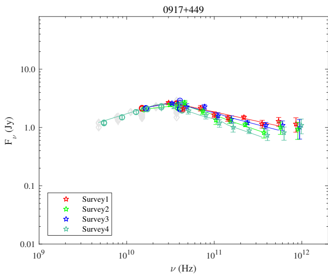
Fig. A.43. 0917+449.
