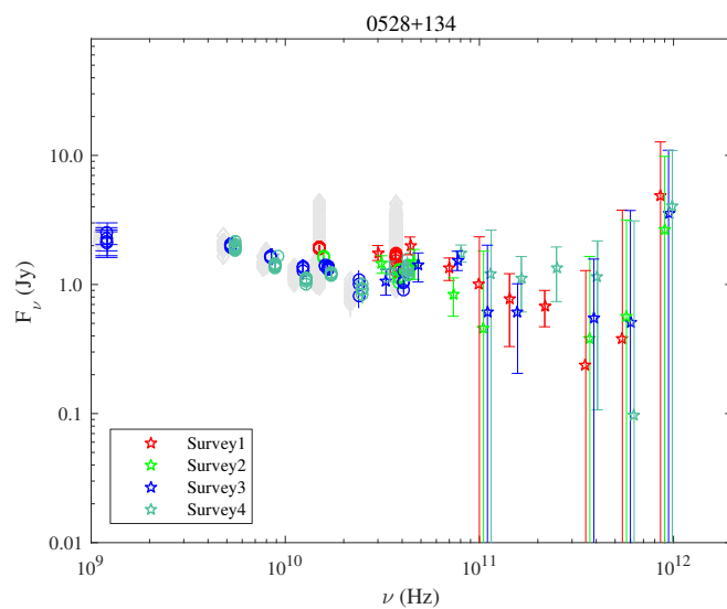
Fig. A.26. 0528+134.
