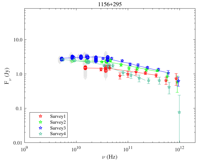
Fig. A.54. 1156+295.
