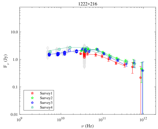
Fig. A.56. 1222+216.
