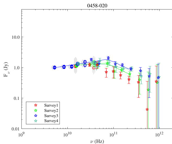
Fig. A.24. 0458-020.
