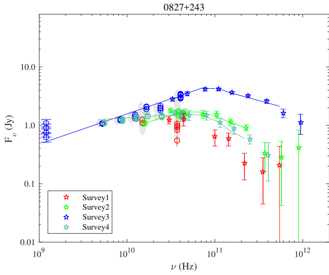
Fig. A.39. 0827+243.
