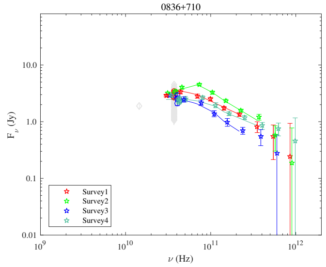
Fig. A.40. 0836+710.
