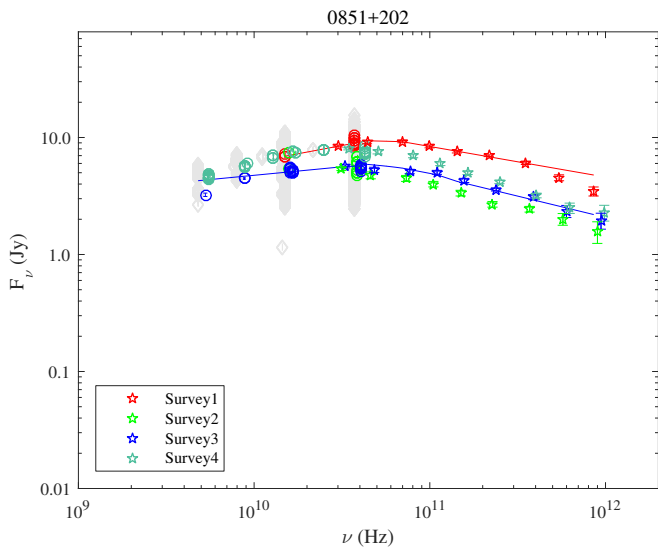
Fig. A.41. 0851+202.
