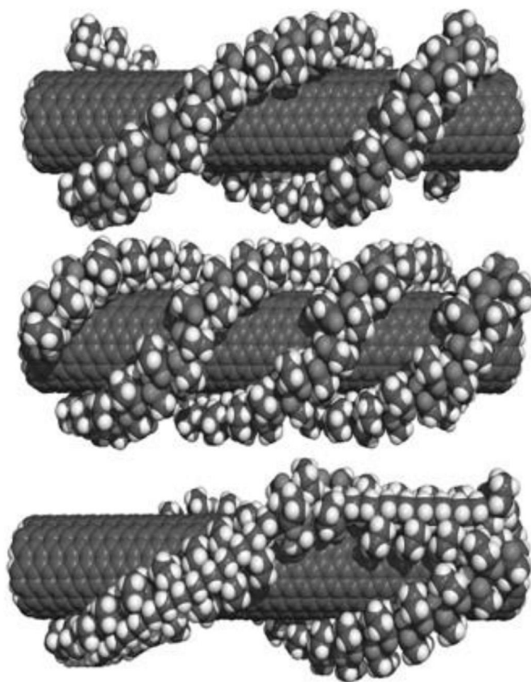
Fig. 12. Examples of polymer wrapping [155].
