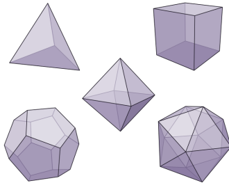
Figura 1. I solidi platonici 1
