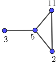
Figura 2. \Delta(M_{11})
